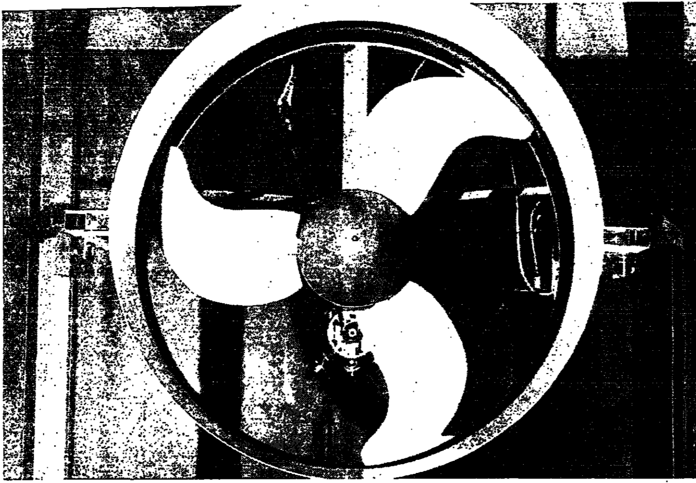
Der neokonstruierte Propeller zeigt, wie man Geräusche, die unter Geräuschentwicklung Luft fördern, leiser machen kann
